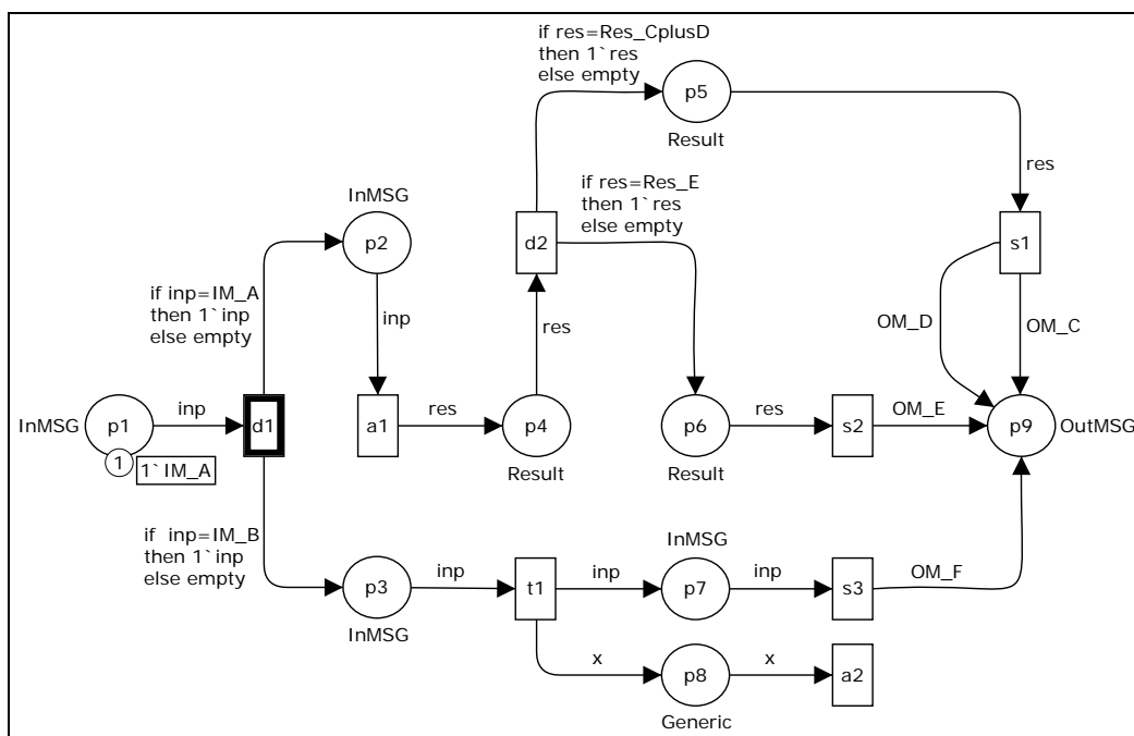
Obr.1 – Ilustrační síť k definici ABA-CPN (zpracováno v nástroji CPN Tools)
